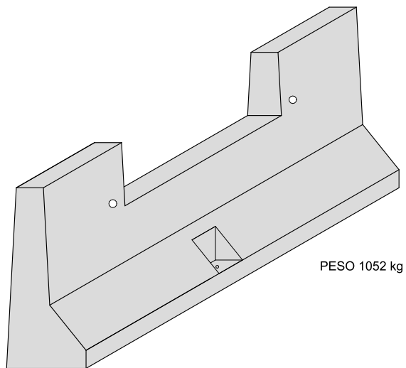
BARRIERA TIPO NEW JERSEY monoscarpa con finestra
