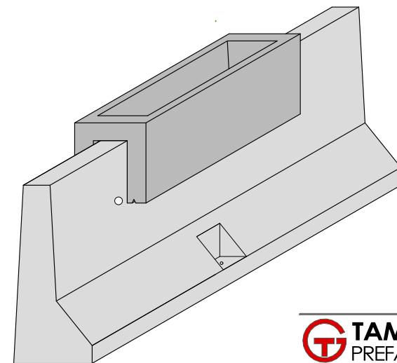
BARRIERA TIPO NEW JERSEY CON FIORIERA ASSEMBLATA SUL POSTO
