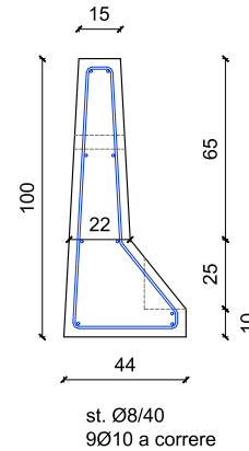
SEZIONE A-A
