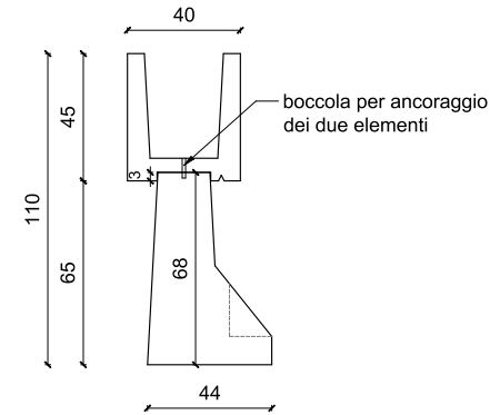
SEZIONE B-B
