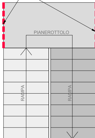
APPOGGIO
