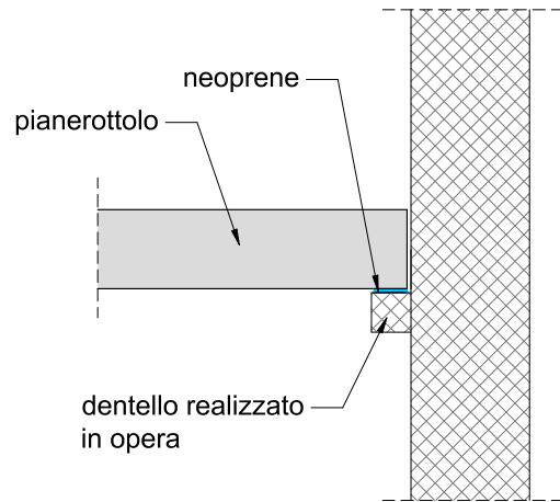
APPOGGIO SEMPLICE
