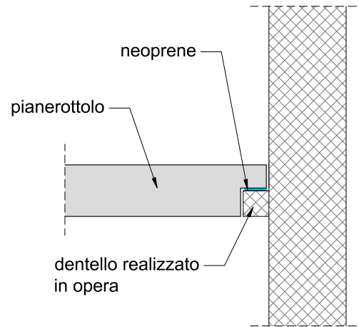
APPOGGIO SEMPLICE con DENTELLO INCASSATO
