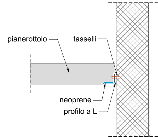
APPOGGIO CON PROFILO A L
