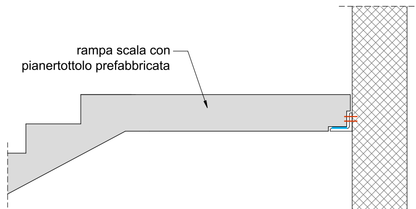
RAMPA+PIANEROTTOLO ANCORATA CON PROFILO A L
