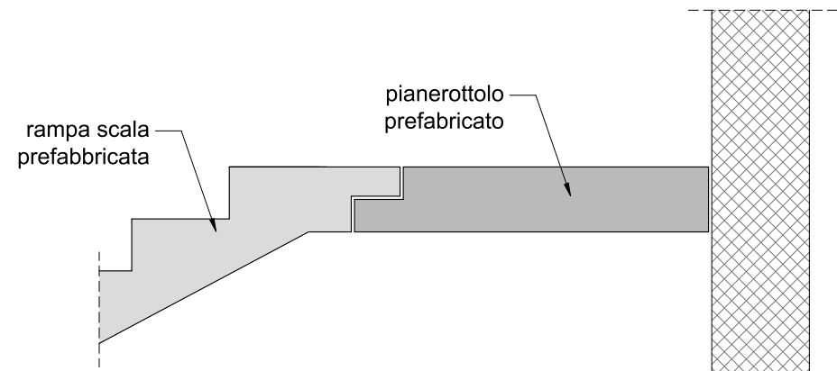
RAMPA CON DENTELLO APPOGGIATA SU PIANEROTTOLO CON DENTELLO
