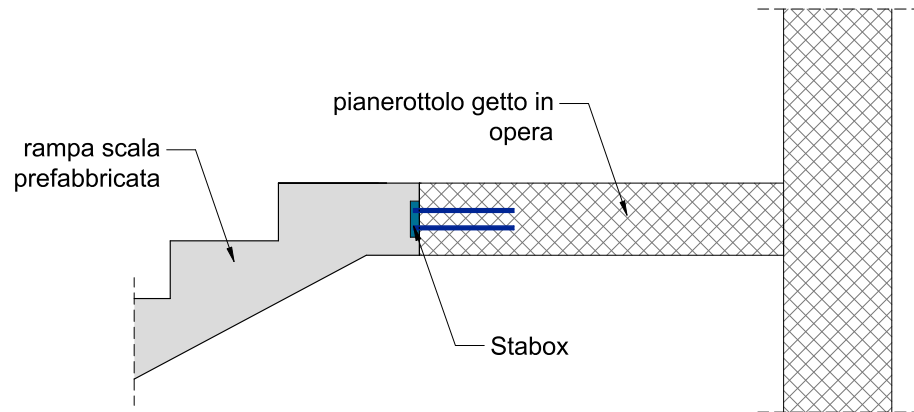
RAMPA CON ACORAGGIO SU PIANEROTTOLO IN OPERA
