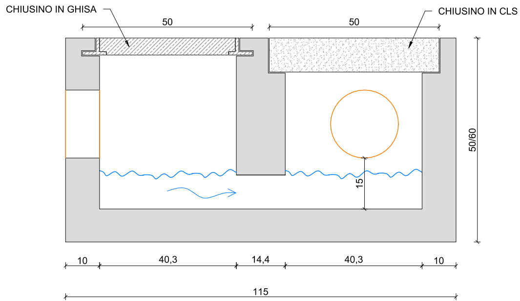
SEZIONE
